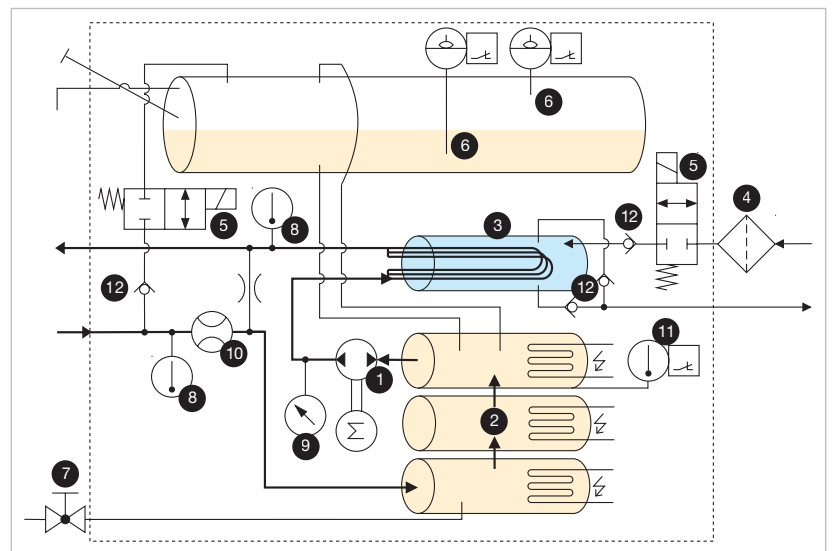
1 Pumpe mit umkehrbarer Pumprichtung, 2 Heizelement, 3 Kühlwendel, 4 Filter, 5 2-2 Wege Ventil (normal geschlossen), 6 Füllstandsensoren, 7 Kugelventil, 8 Temperaturfühler, 9 Drucksensor, 10 Durchflusssensor, 11 Sicherheitstemperaturbegrenzer, 12 Rückschlagventil
